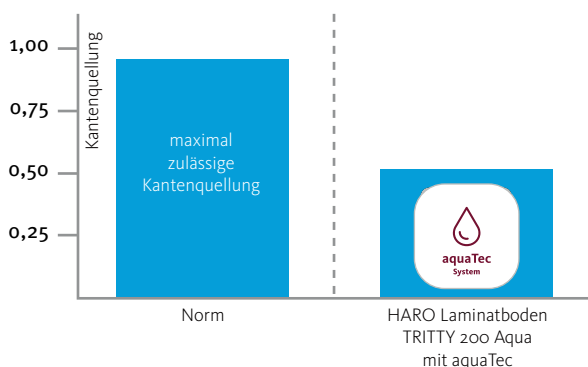
Kantenquellung von Laminatböden bei Wassereinfluss
